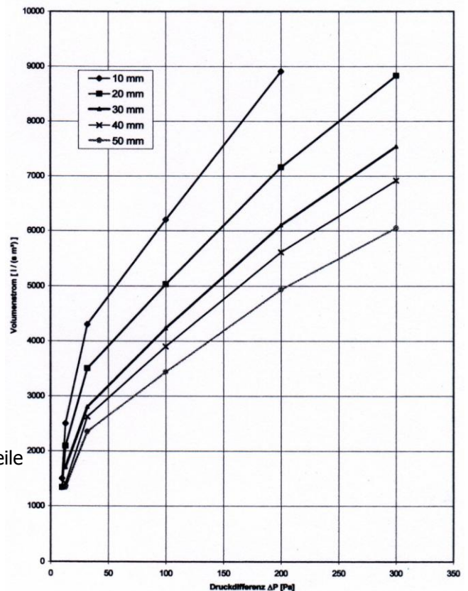
Luftwiderstandskurve PPI 10
