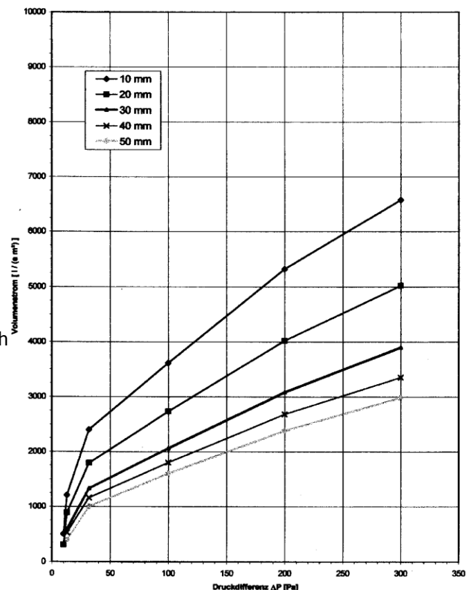
Luftwiderstandskurve PPI 30
