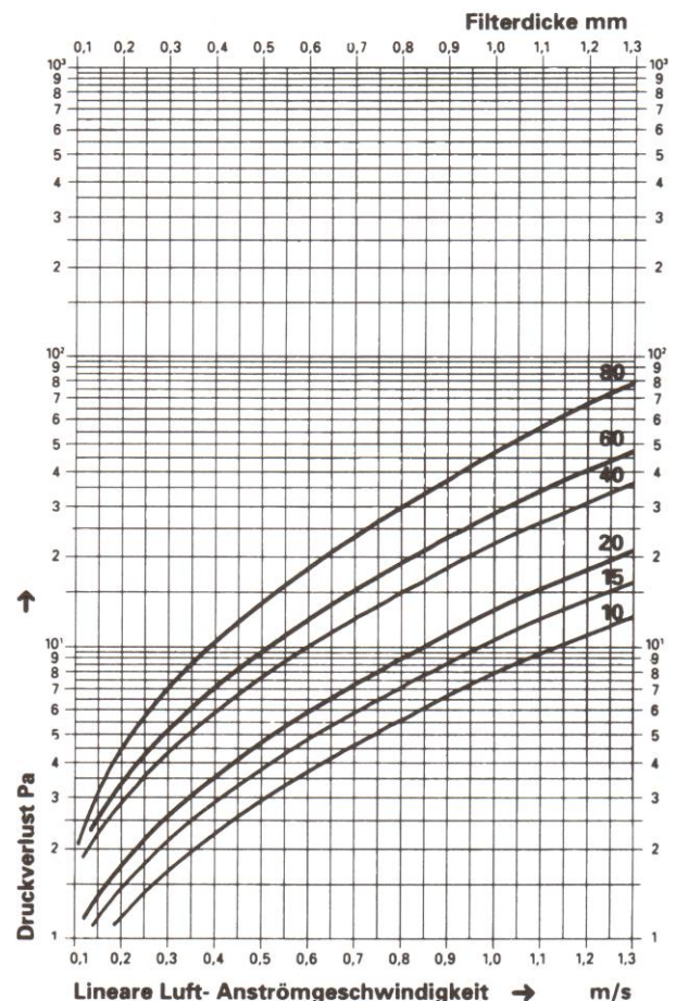
Luftwiderstandskurve PPI 30 Ä
